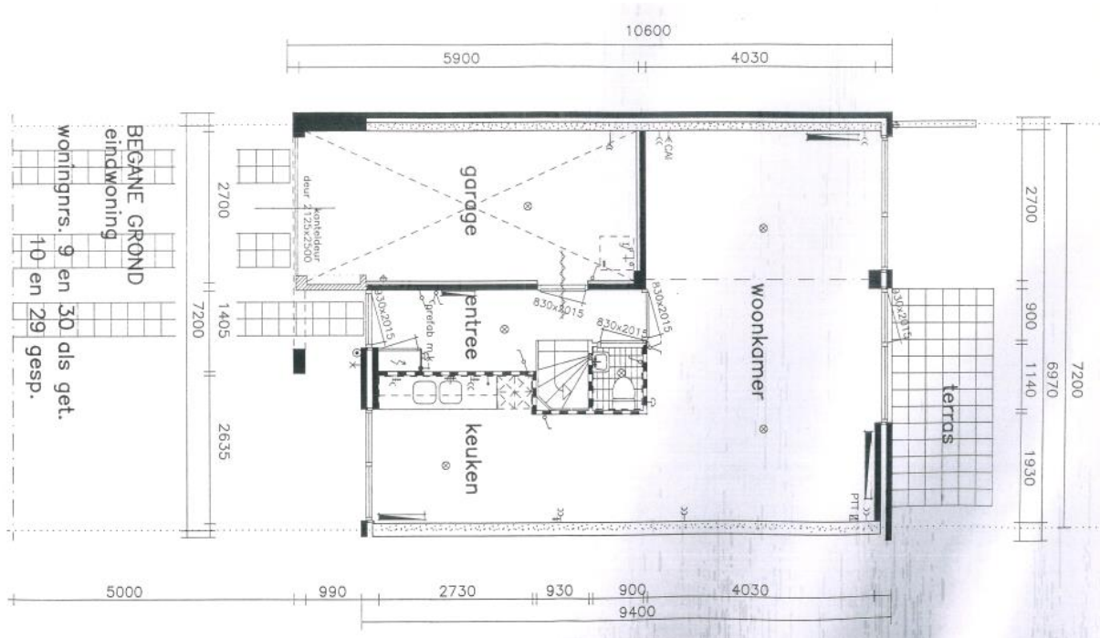
Figuur 2 (Begane grond woningen Kramerstraat)
